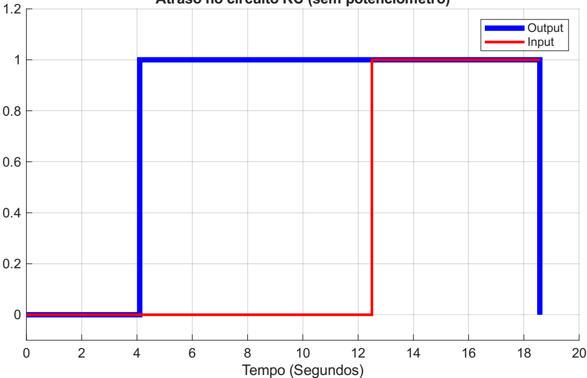
Atraso no circuito RC (sem potenciômetro)
